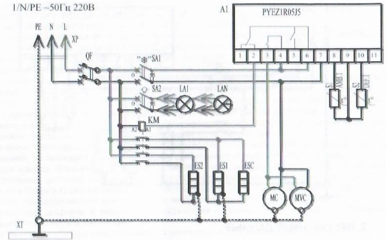
Рис.4. Схема электрическая принципиальная витрины холодильной ВХСн-0,94 (1,25) Carboma GC110.
