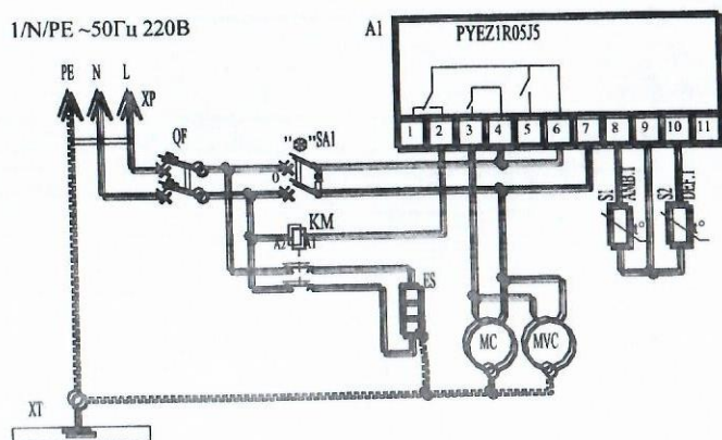
Рис.6. Схема электрическая принципиальная витрины холодильной ВХСо-0,94 (1,25; 1,5; 2,0); ВХСл-0,94 (1,25; 1,5; 2,0) Carboma GC110.
