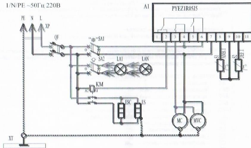
Рис.2. Схема электрическая принципиальная витрины холодильной ВХСр-0,94 (1,25; 1,5; 2,0) Carboma GC110.
