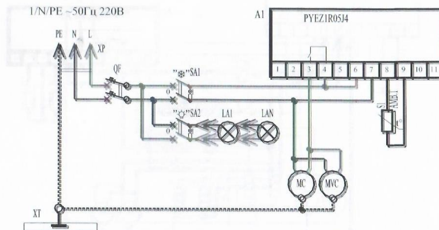
Рис.1. Схема электрическая принципиальная витрины холодильной ВХС-0,94 (1,25; 1,5; 2,0; 2,5) Carboma GC110.
