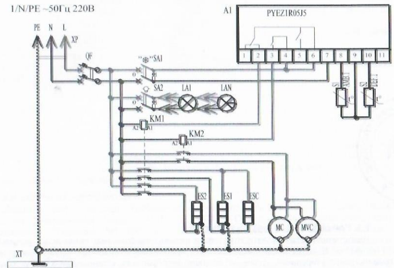
Рис.5. Схема электрическая принципиальная витрины холодильной ВХСн-1,5 (2,0) Carboma GC110.
