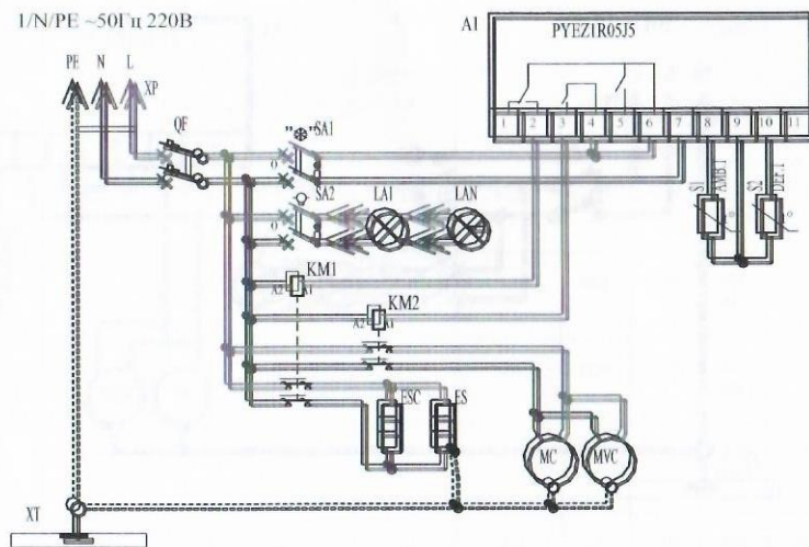
Рис.3. Схема электрическая принципиальная витрины холодильной ВХСр-2,5 Carboma GC110.
